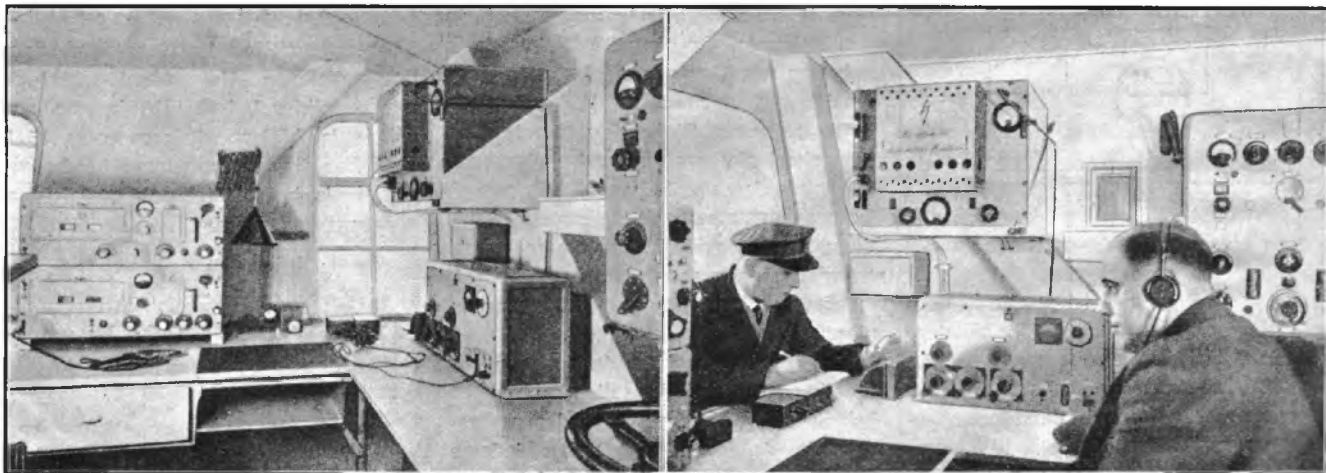
DE RADIO-CABINE VAN DE „GRAF ZEPPELIN”
